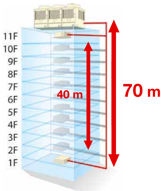
Max. převýšení mezi venkovní jednotkou a poslední vnitřní jednotkou
