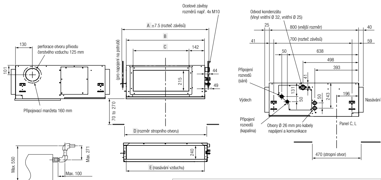
Dimenzování odvodu kondenzátu
